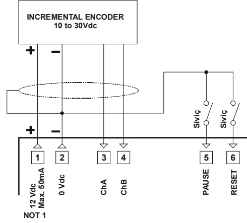
DIP SİVİÇ AYARI : NPN Incremental Encoder & sviç bağlantısı
