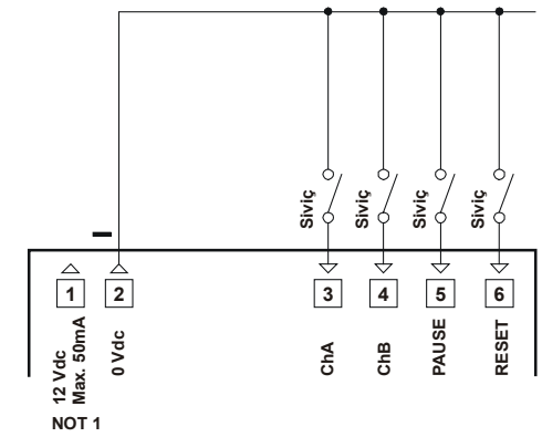
DIP SİVİÇ AYARI : NPN Sviçbağlantısı
