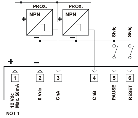
DIP SİVİÇ AYARI : NPN Proximity & sviç bağlantısı
