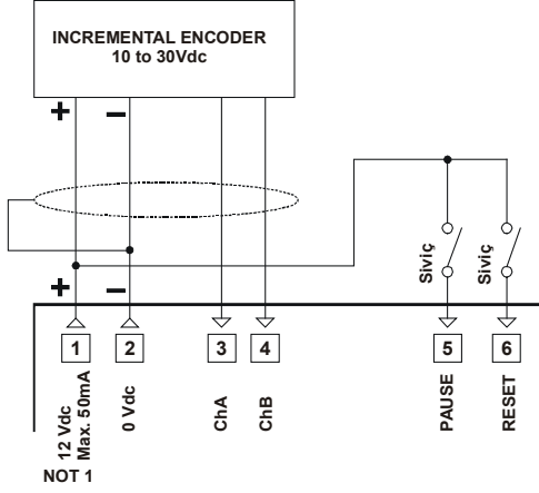
DIP SİVİÇ AYARI : PNP Incremental Encoder & sviç bağlantısı
