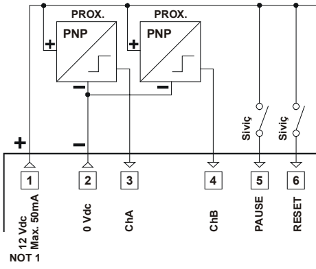
DIP SİVİÇ AYARI : PNP Proximity & sviç bağlantısı
