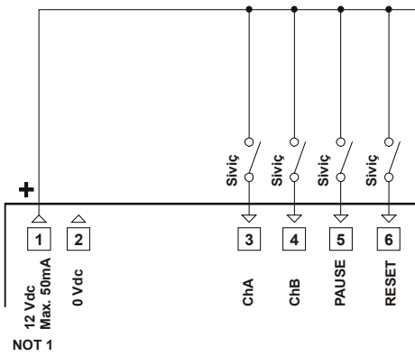
DIP SİVİÇ AYARI : PNP Sviçbağlantısı
